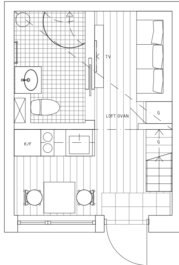
Entréplan, skala 1:50.
