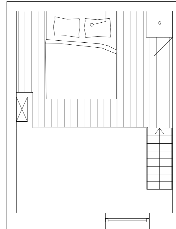
Loftplan, skala 1:50.
